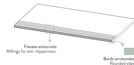
BORDO ANTISCIVOLO ANTI-SKID EDGE
