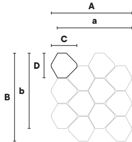
A 33,2 cm / 13" a 30,5 cm / 12" B 36 cm / 14" b 30,8 cm / 12" C 10,6 cm / 4" D 10,1 cm / 4"
