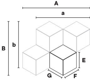
A 44,2 cm / 18" B 35,6 cm / 14" a 35,2 cm / 14" b 30,5 cm / 12" E 10 cm / 4" F 8,66 cm / 4" G 10 cm / 4"
